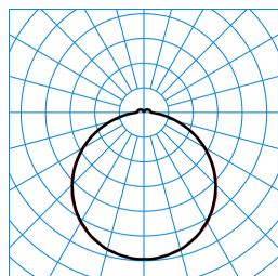
Olisq QWD3 DW 45-830 ET HFS IP54 IK + Olisq QWD3 ZDR 1/2 03 TX461274 ■ C0 - C180 ■ C90 - C270
