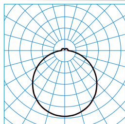
Olisq QWD3 DW 45-830 ET HFS IP54 IK TX778296 ■ C0 - C180 ■ C90 - C270
