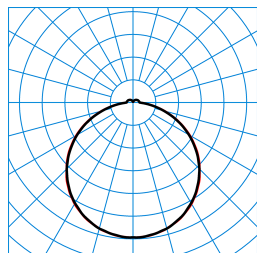
Olisq QWD3 DW 45-830 ET HFS IP54 IK + Olisq QWD3 ZDR 1/2 01 TX460881 ■ C0 - C180 ■ C90 - C270
