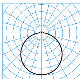
Olisq QWD3 DW 45-830 ET HFS IP54 IK + Olisq QWD3 ZDR 1/2 05 TX461711 ■ C0 - C180 ■ C90 - C270
