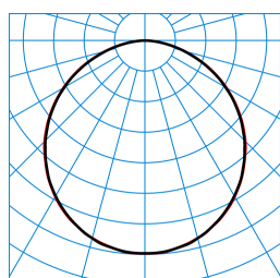
Olisq QWD3 DW 45-830 ET HFS IP54 IK + Olisq QWD3 ZDR 1/1 01 TX461729 ■ C0 - C180 ■ C90 - C270
