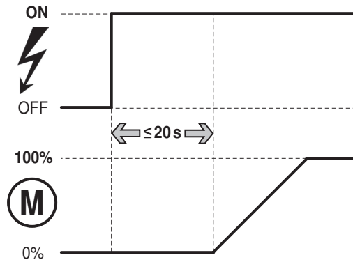
MF40ER-24M
