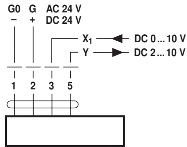
MF40ER-24M
