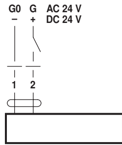
MF40ER-24T
