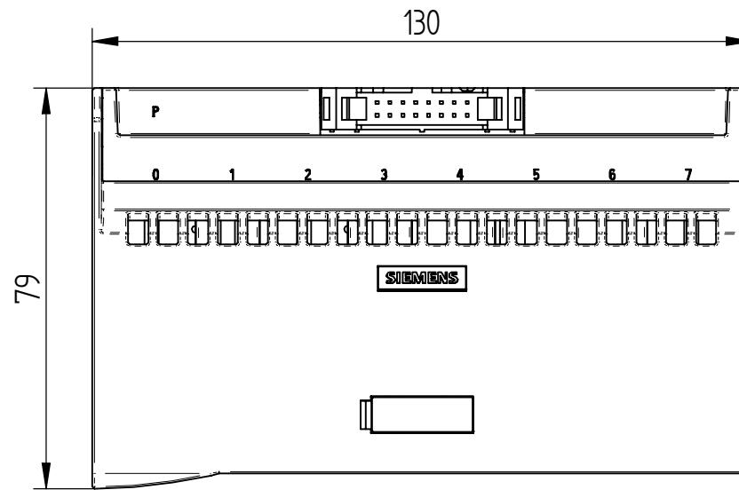
Vorne / Front
