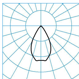
SNS ACT-SUM RC7-HR1VFL-26 ■ C0 - C180
