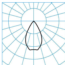
SNS ACT-CW RC7-HR1VFL-26 ■ C0 - C180
