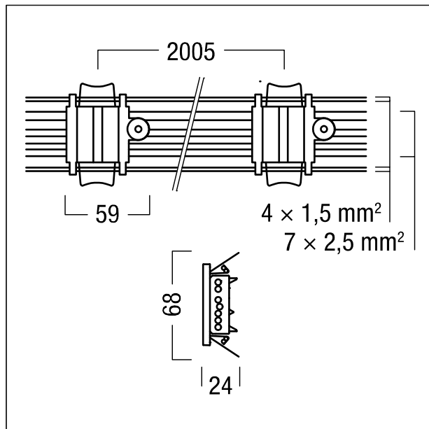
ZS_TRS_M_Verdrahtung_11pol_2000.wmf
