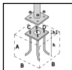
S.2849 Embase de fixation à sceller pour POTEAU S.2801, S.2813, S.2843, S.2845
