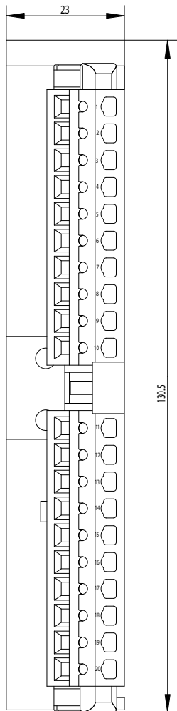
Vorne / Front
