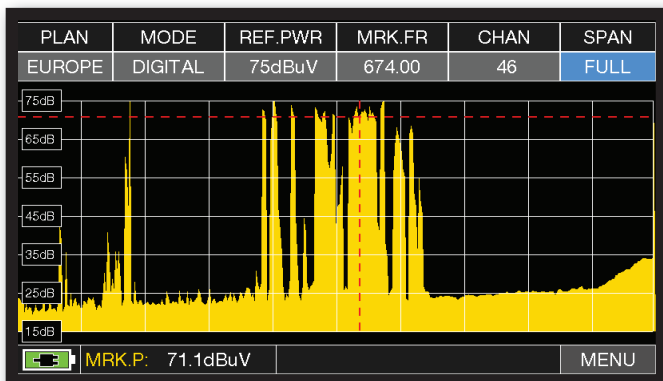
Spectre COMPLET « TV » (de 5 à 1.250 MHz).
