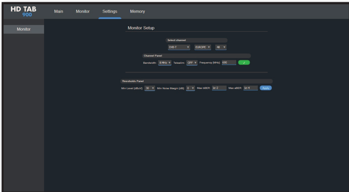
Exemple de RÉGLAGE d'un CANAL DE RÉCEPTION TV (Norme DVB-T) et les SEUILS D'ALARME (SEUILS) correspondants
