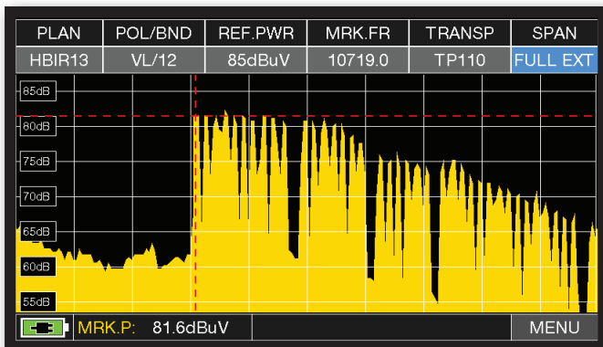
Spectre « SAT » SPAN FULL EXT (de 230 à 2610 MHz) avec un LNB universel.
