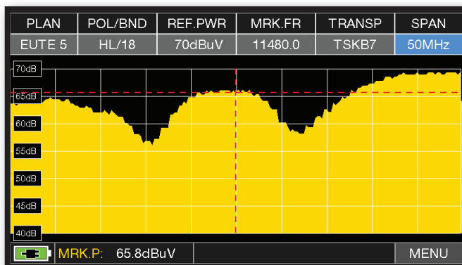
Visualisation d'un transpondeur SCPC (programmes non multipléxés) avec paramétrage : « FILTRE RBW 5 MHz » et « dB DIV 5dB » (Span 50 MHz)
