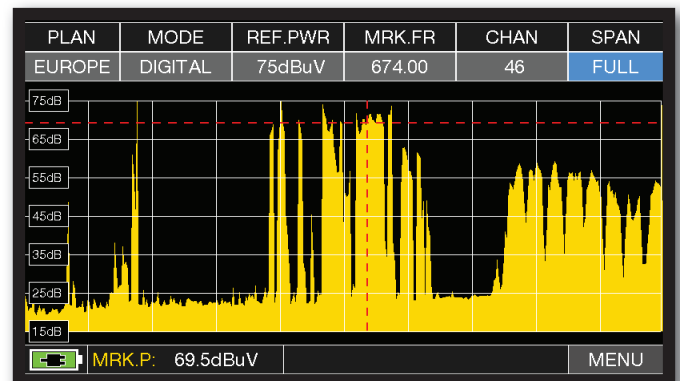
TV SPAN FULL spectre avec signaux SAT de canaux mixtes (de 5 à 1.250 MHz).
