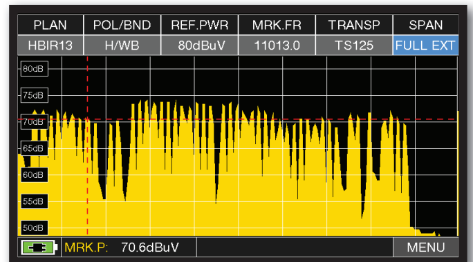
Spectre « SAT » SPAN FULL EXT (de 230 à 2610 MHz) avec un LNB LARGE BANDE.
