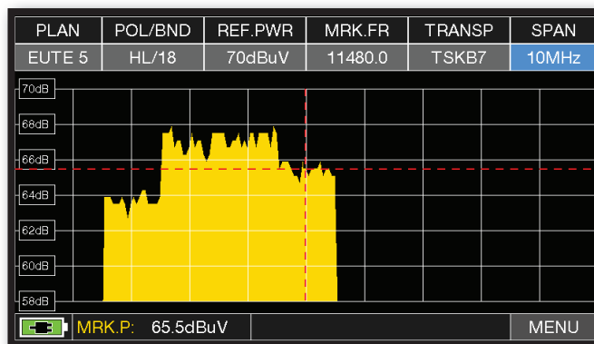
Visualisation d'un transpondeur SCPC (programmes non multipléxés) avec paramétrage : (SPAN 10 MHz).
