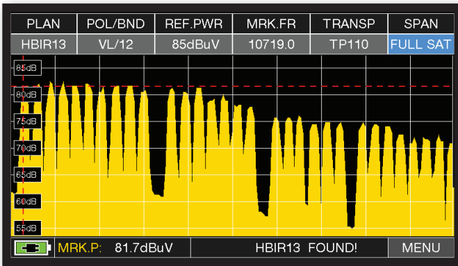
Spectre SAT SPAN (zoom) FULL SAT (de 930 à 2250 MHz).
