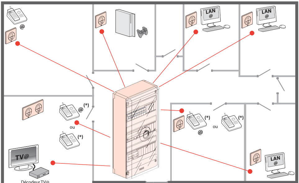
Sortie de câble
