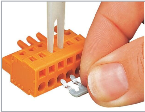
Outil de manipulation pour montage du peigne de pontage 231-902
