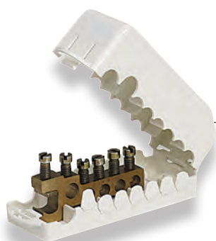
Répartiteur de terre 5 dérivations (Q100)
