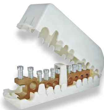
Répartiteur de terre 8 dérivations (Q130)
