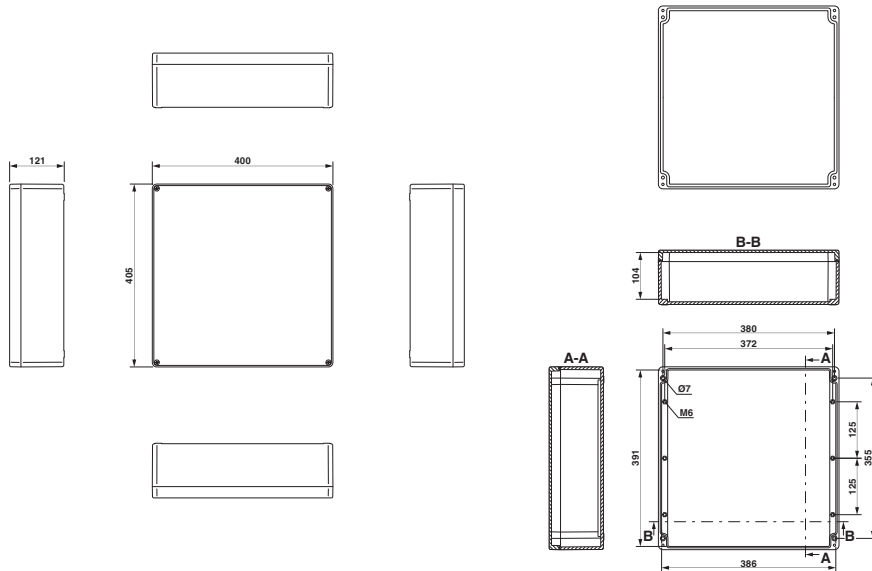
Dessin coté
