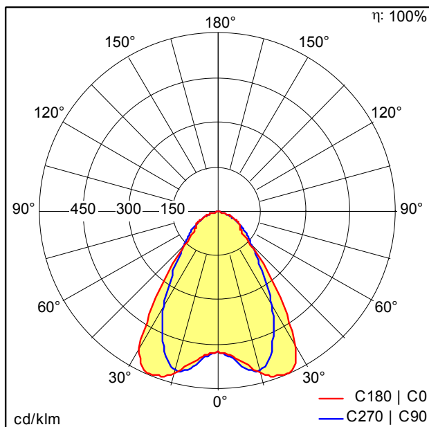
D44421AA_TEC_LED16000-840_L2000_WB_LDE_WH_IP.idt
