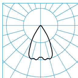
InperiaLP C05 HR22 2700-830 03 + RD-PC ■ C0 - C180 TX373864
