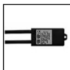
S.2407 ALIMENTATION ELECTRONIQUE NON GRADABLE 14,4W 230Vac/24Vdc IP67 Entrée: 230V Courant alterné Sortie: 24V Courant continu. Le nombre maximum d'appareils dépend de la somme des puissances unitaires de l'appareil. IP67 CLASSE II SELV Dimensions: 79 x 38 x 25 mm L'UTILISATION DU DÉCHARGEUR À SURTENSION S.2499 EST RECOMMANDÉE POUR CHAQUE BALLAST ÉLECTRONIQUE QUI DOIT ÊTRE INSTALLÉ À UNE DISTANCE MAXIMALE DE 10m DE CELUI-CI.
