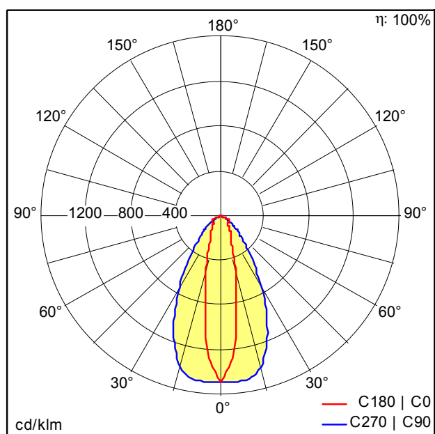
D44423AA_TEC_LED5500-840_L1500_NB_LDE_SR_IP.lct
