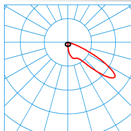
LnStar 70-AM1R-LRA/20000-740 6G2C TX051201 ■ C0 - C180 ■ C90 - C270 DIN 5040: A30 UTE: 1,00 l CEN Flux Code: 25 70 98 100 100
