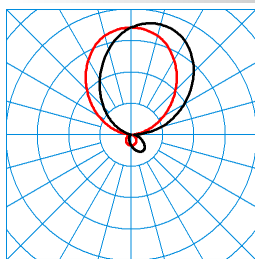
Sanesca W3 LED5000-830 03 TX050874 ■ C0 - C180 ■ C90 - C270 DIN 5040: D33 UTE: 0,12 E + 0,88 T CEN Flux Code: 43 75 93 12 100 50 80 96 88
