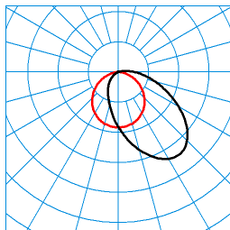
Sanesca W3 LED5000-830 03 (reading light) TX055767 ■ C0 - C180 ■ C90 - C270 DIN 5040: A30 UTE: 0,98 E + 0,02 T CEN Flux Code: 43 75 93 98 100 9 22 30 2
