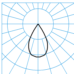
E-Line 7751 B.VEO RFS-VFL 05 30-BC J24 ETDD L37 01 ■ C0 - C180 TX095122
