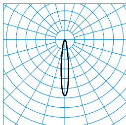
E-Line 7751 B.VEO RFS-SP 05 30-BC J24 ETDD L37 01 ■ C0 - C180 TX095606
