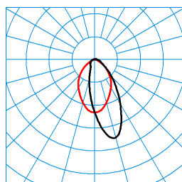
TX064312 DIN 5040: A50 UTE: 0,97 C + 0,03 T C0 - C180 C90 - C270
