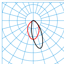
TX064313 DIN 5040: A50 UTE: 0,97 C + 0,03 T C0 - C180 C90 - C270
