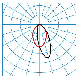
TX064311 DIN 5040: A50 UTE: 0,97 C + 0,03 T C0 - C180 C90 - C270
