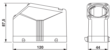
Dessin coté
