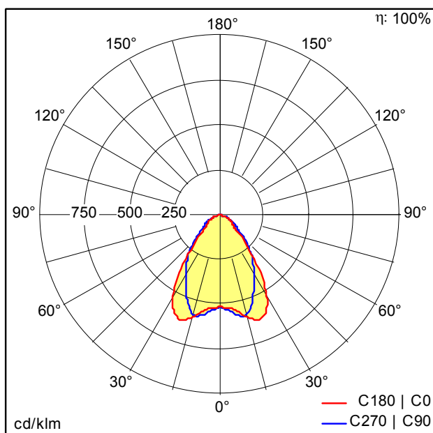
D35001AA_TECTON_C_LED5500-865_L1500_WB_LDE_SR.Idt
