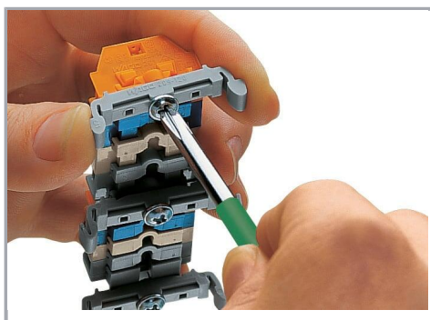
Barrettes à bornes ; avec brides de fixation,
