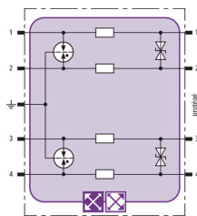
Schéma de principe du circuit BXT ML4 BD 12
