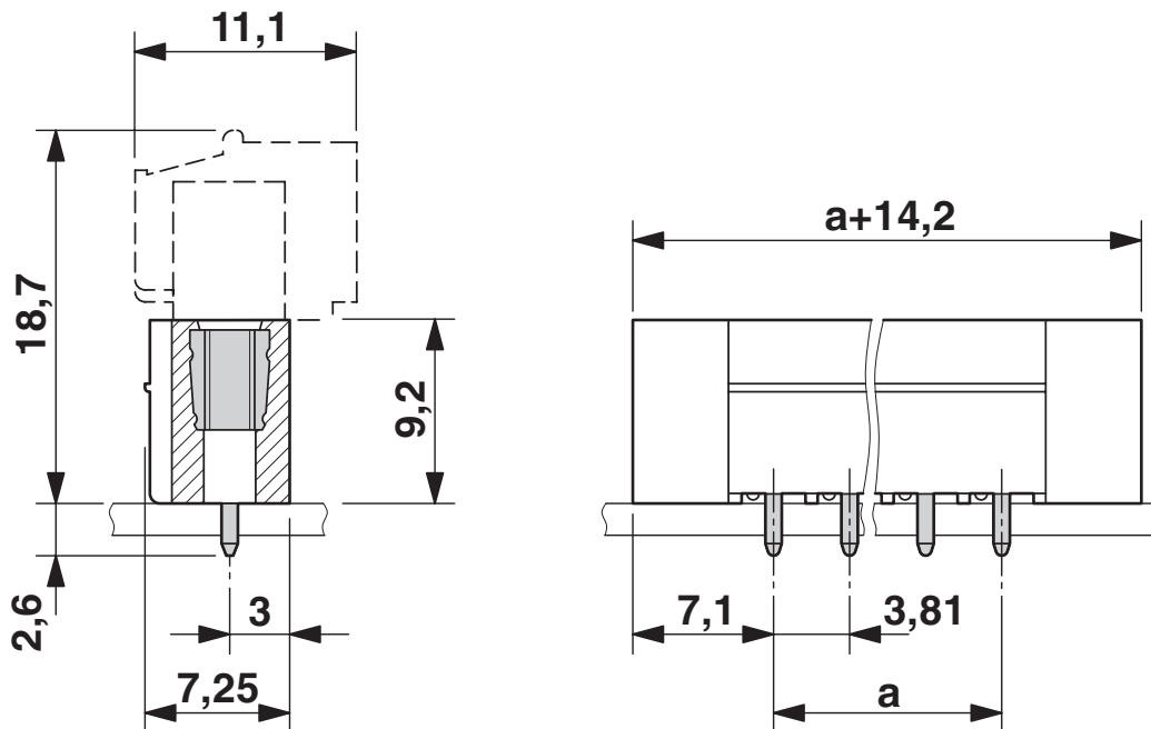
Dessin coté
