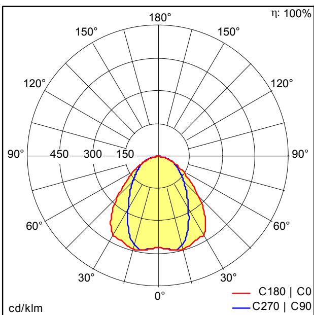
D44422AA_TEC_LED5200-840_L1000_VWB_LDE_SR_IP.ltd
