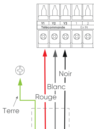
Câble de la télécommande
