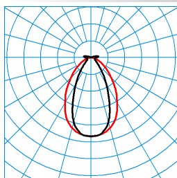
AragFHE 15 PN 80-840 PC LHT TX194646
