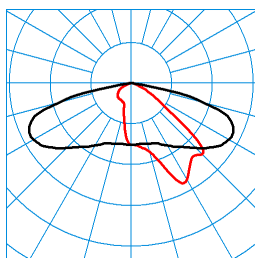
Jovie 50-AB2L-ML/4600-6800-730 6G1 ETDD (CLO initial value) TX271470 ■ C0 - C180 ■ C90 - C270 DIN 5040: A30 UTE: 1,00 G CEN Flux Code: 35 71 96 100 100
