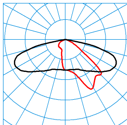
Jovie 50-AB2L-ML/4600-6800-730 6G1 ETDD (5600 lm) TX068688 ■ C0 - C180 ■ C90 - C270 DIN 5040: A30 UTE: 1,00 G CEN Flux Code: 35 71 96 100 100
