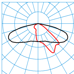
Jovie 50-AB2L-ML/4600-6800-730 6G1 ETDD (6800 lm) TX068689 ■ C0 - C180 ■ C90 - C270 DIN 5040: A30 UTE: 1,00 G CEN Flux Code: 35 71 96 100 100
