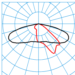
Jovie 50-AB2L-ML/4600-6800-730 6G1 ETDD (CLO end value) TX271468 ■ C0 - C180 ■ C90 - C270 DIN 5040: A30 UTE: 1,00 G CEN Flux Code: 35 71 96 100 100
