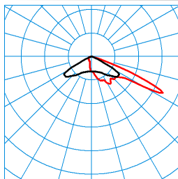
LnPlus 70-AM19L-SLR1/62000-730 48G1 ET (CLO end value) TX376948 ■ C0 - C180 ■ C90 - C270 DIN 5040: A30 UTE: 1,00 J CEN Flux Code: 28 76 99 100 100
