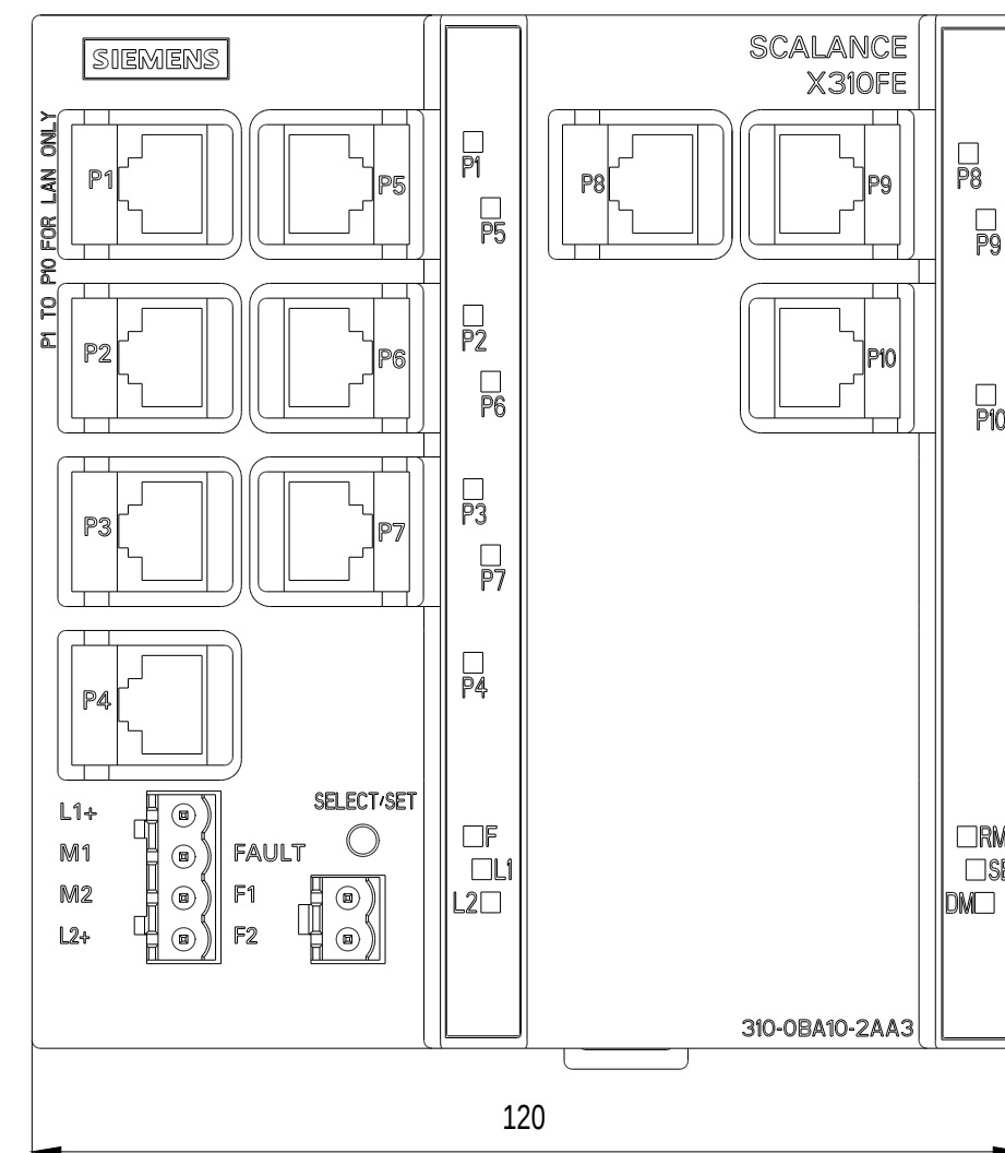
Vorne / Front
