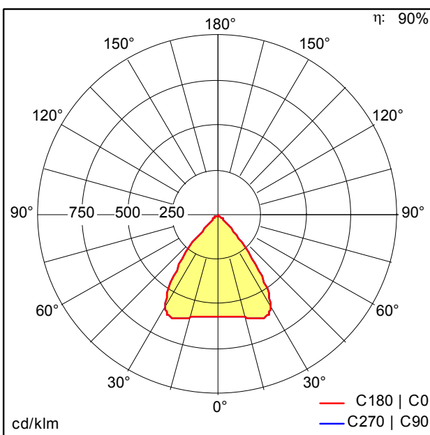
ST7965_N.Idt
