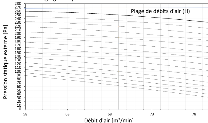
Caractéristiques du ventilateur (2)
