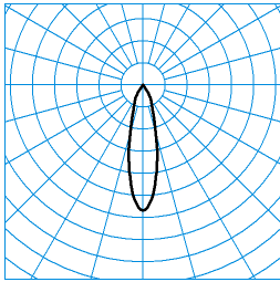
E-Line 7751 B.VEO RFS-MF 05 20-EW J10 ET L37 05 ■ C0 - C180 TX095344
