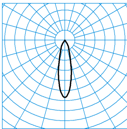
E-Line 7751 B.VEO RFS-MF-c 05 20-EW J10 ET L37 05 ■ C0 - C180 TX095443
