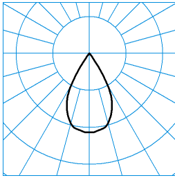
E-Line 7751 B.VEO RFS-VFL-c 05 20-EW J10 ET L37 05 ■ C0 - C180 TX095796
