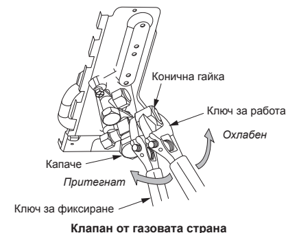
Клапан от газовата страна
