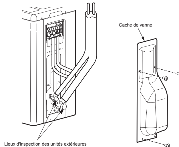
Lieux d'inspection des unités extérieures
