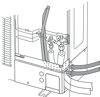
Connexion latérale
