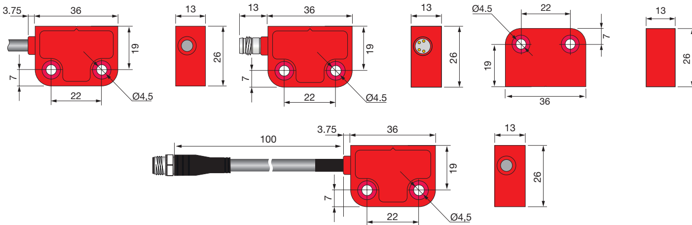
Fig. 1 - Dimensions
