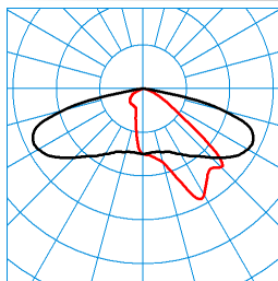
Jovie 50-AB2L-LRA/1800-740 4G1 ET TX076473 ■ C0 - C180 ■ C90 - C270 DIN 5040: A30 UTE: 1,00 G CEN Flux Code: 34 71 96 100 100
