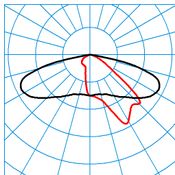
Jovie 50-AB2L-LRA/1800-740 4G1 ET (CLO end value) TX301570 ■ C0 - C180 ■ C90 - C270 DIN 5040: A30 UTE: 1,00 G CEN Flux Code: 34 71 96 100 100
