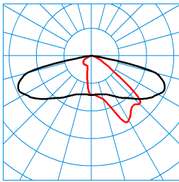
Jovie 50-AB2L-LRA/1800-730 2G1 ET TX068558 ■ C0 - C180 ■ C90 - C270 DIN 5040: A30 UTE: 0,98 l CEN Flux Code: 34 70 96 100 98
