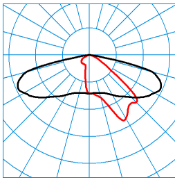
Jovie 50-AB2L-LRA/1800-730 2G1 ET (CLO initial value) TX301084 ■ C0 - C180 ■ C90 - C270 DIN 5040: A30 UTE: 0,98 l CEN Flux Code: 34 70 96 100 98
