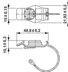
Dessin coté
