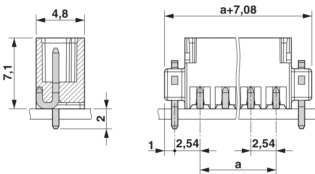
Dessin coté
