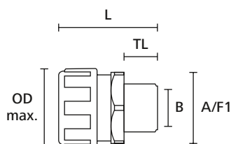
Raccord droit HelaGuard avec filetage externe fixe
