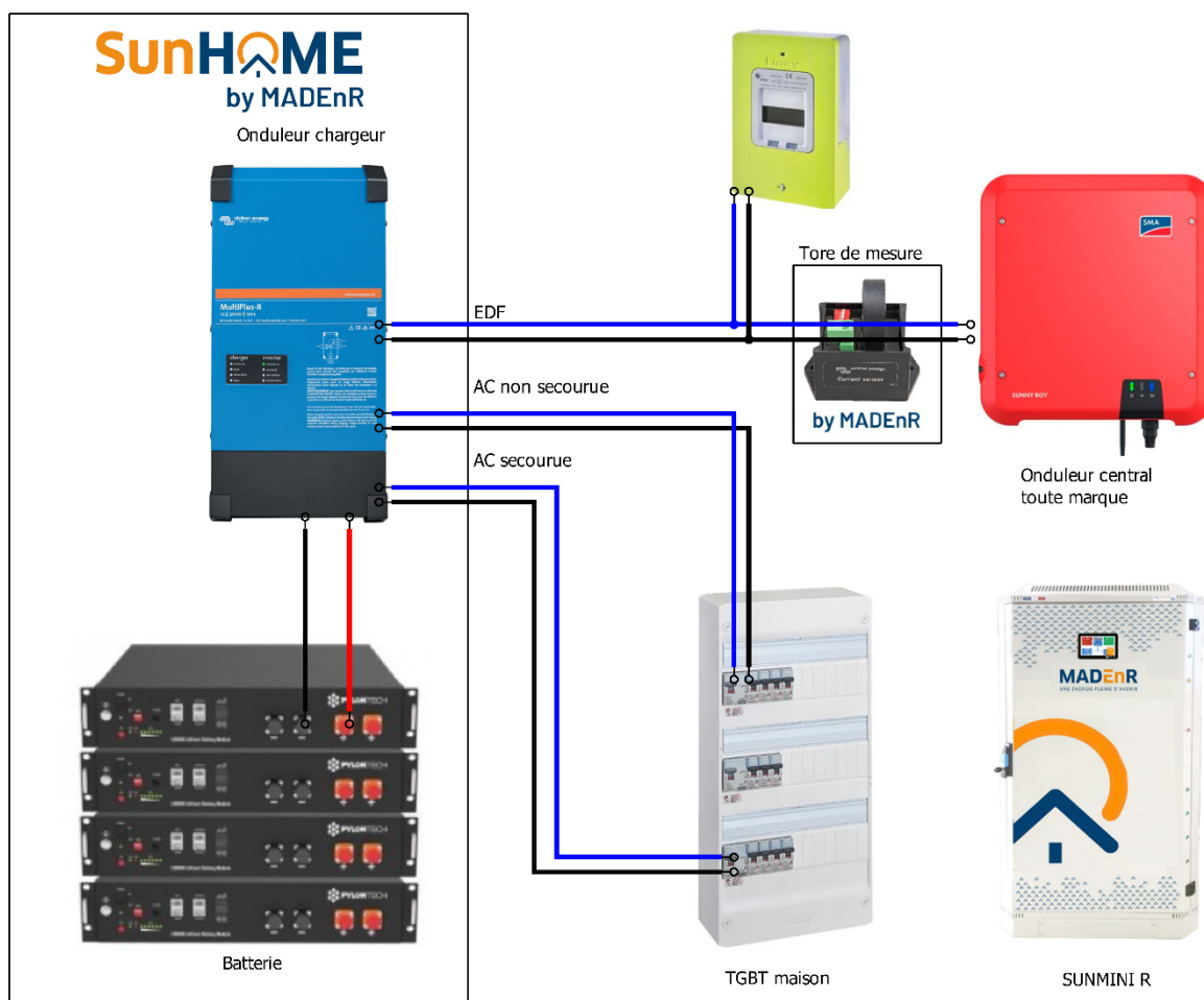
Figure 51 : Schéma de principe de la SunMini R
