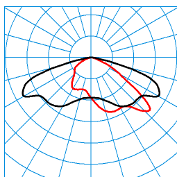
Jovie 70-AB7L-ML-LR/165-240-740 24G1 ET (CLO initial value) TX271479 ■ C0 - C180 ■ C90 - C270 DIN 5040: A30 UTE: 1,00 G CEN Flux Code: 35 73 97 100 100
