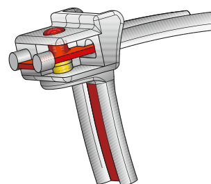
Le collier est verrouillé grâce au pion, qui vient déformer la matière.
