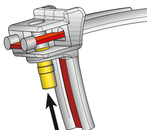
Tête d'un collier KR avant verrouillage.
