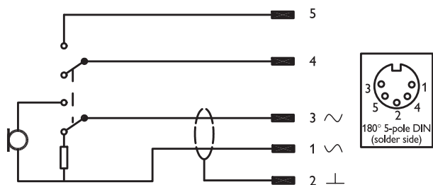
Diagramme électrique
