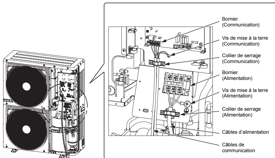
Le couvercle du boîtier de commande électrique
