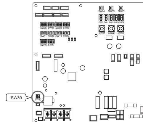
Cartes de circuits imprimés de l'interface de l'unité principale
