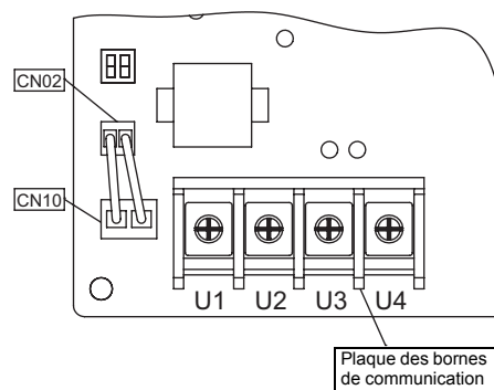
[U1, U2] et [U3, U4] raccordés
