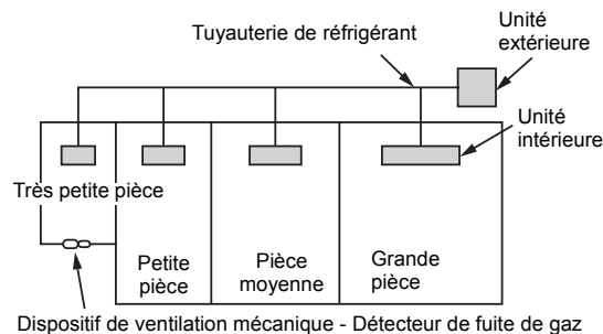
Dispositif de ventilation mécanique - Détecteur de fuite de gaz
