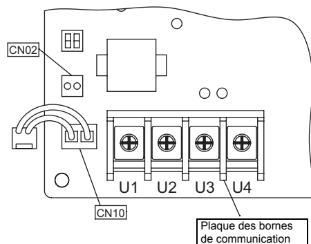
[U1, U2] et [U3, U4] non raccordés
