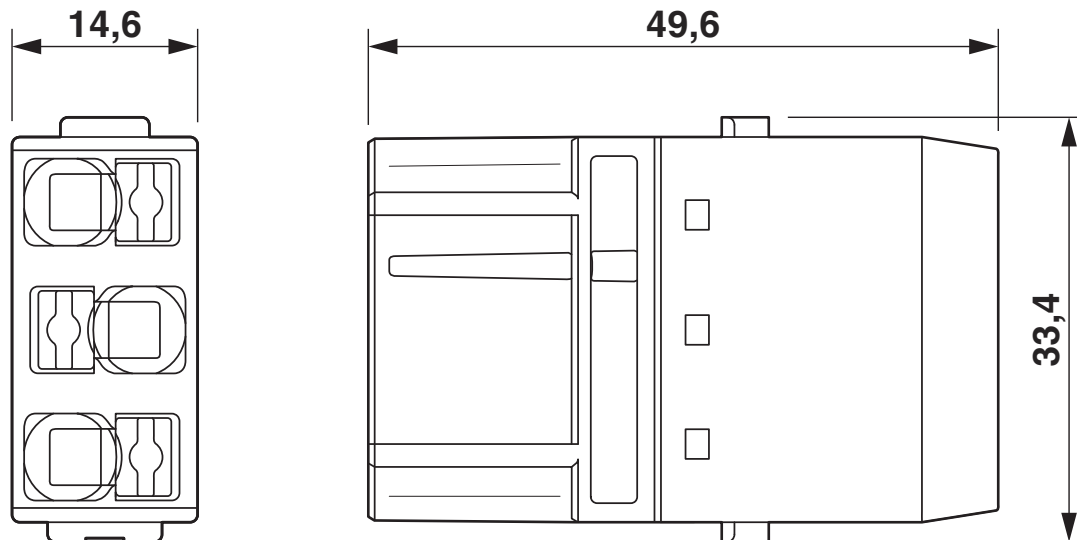
Dessin coté
