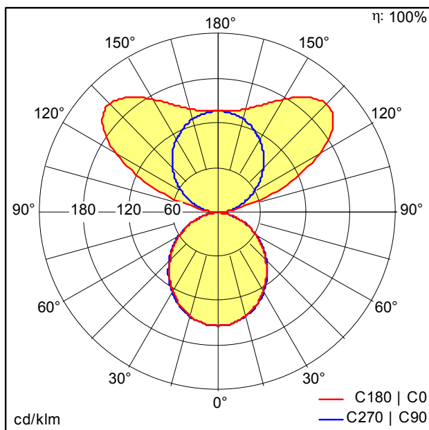
D42843AA+D44969AA_SLOIN_SLIM_ID_840_L1750_PC_SR.Idt
