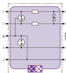
Schéma de principe du circuit BXT ML2 BD S 12
